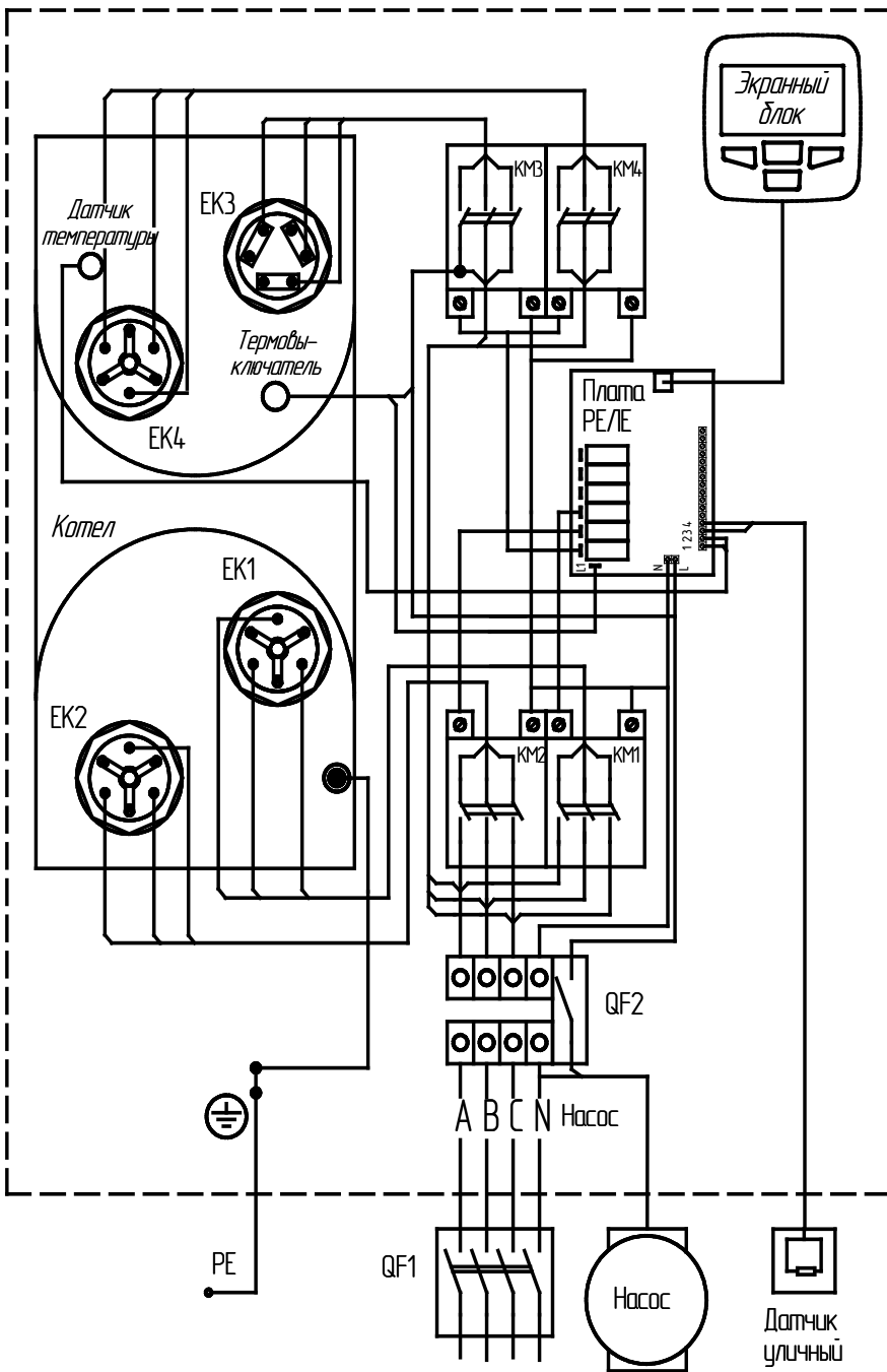
Рисунок 5. Схема подключения ZVAN UNIVERSAL -36 - 11 -
